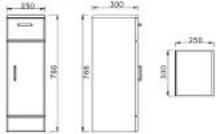
CG30D Cabinet: 250 x 300 x 766mm
