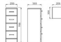
CG30D(4CT) Cabinet: 250 x 300 x 766mm
